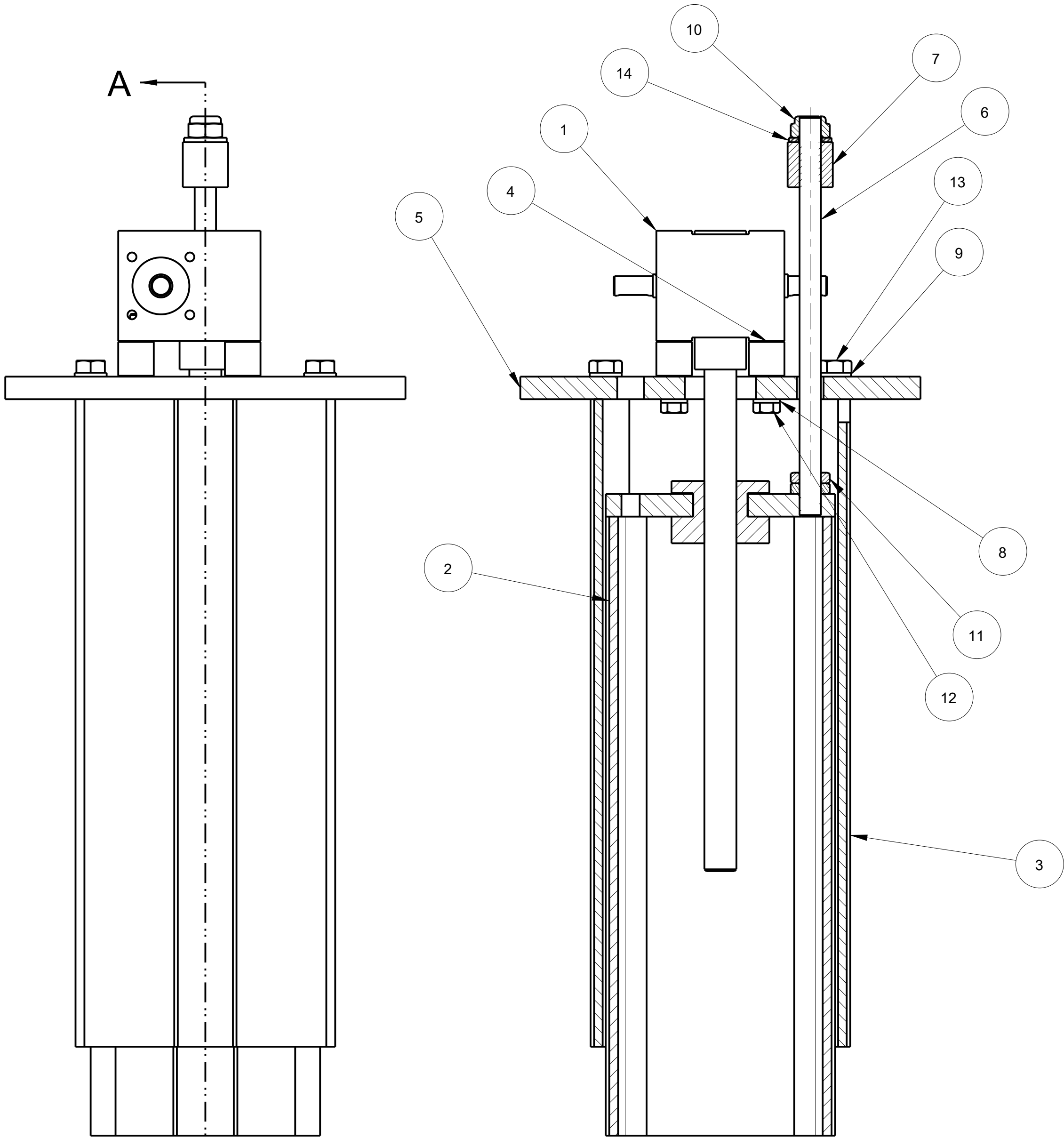
SECTION A-A
